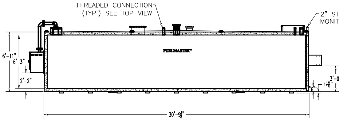
ELEVATION
